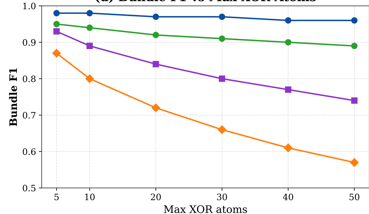
(d) Bundle F1 vs Max XOR Atoms
